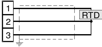
Fig. 5 Connexion de thermorésistance
