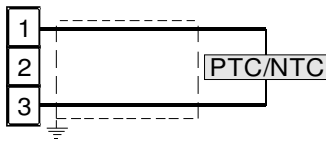
Fig. 6 Connexion de thermisteur
