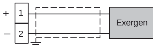
Fig. 4 - Câblage du capteur à infrarouge
