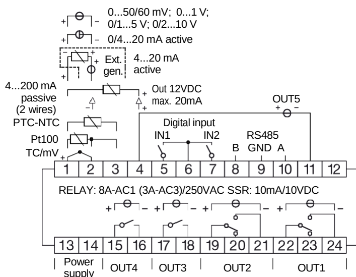
Fig. 2 - Connexions électriques
