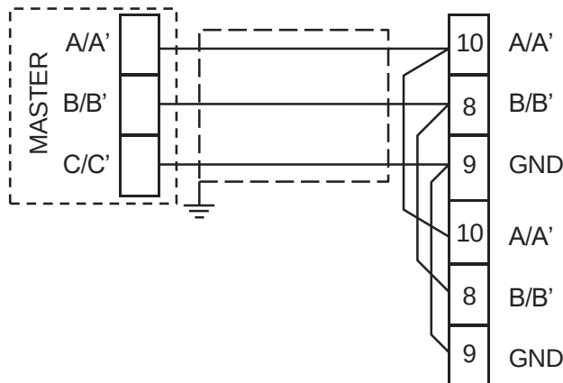
Fig. 11 - Câblage de l'interface de communication série
