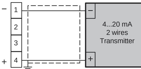
Fig. 8 - Câblage de signaux en 0/4... 20 mA à transmetteur passif avec alimentation auxiliaire
