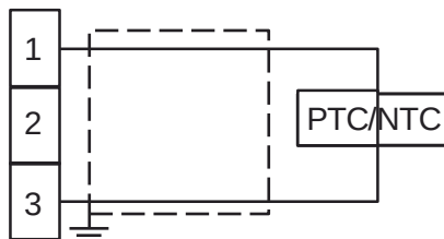
Fig. 6 - Câblage pour PTC/NTC
