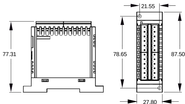
Fig. 1 - Dimensions du contrôleur
