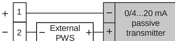
Fig. 9 - Câblage de signaux en 0/4... 20 mA à transmetteur passif avec alimentation externe
