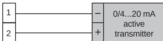
Fig. 10 - Câblage de signaux en 0/4... 20 mA à transmetteur actif
