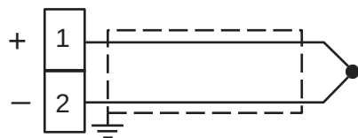
Fig. 3 - Connexion des thermocouples
