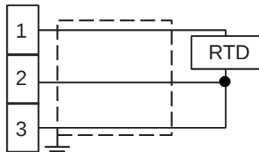
Fig. 5 - Connexion de thermorésistance
