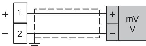
Fig. 7 - Câblage pour signaux en V/mV
